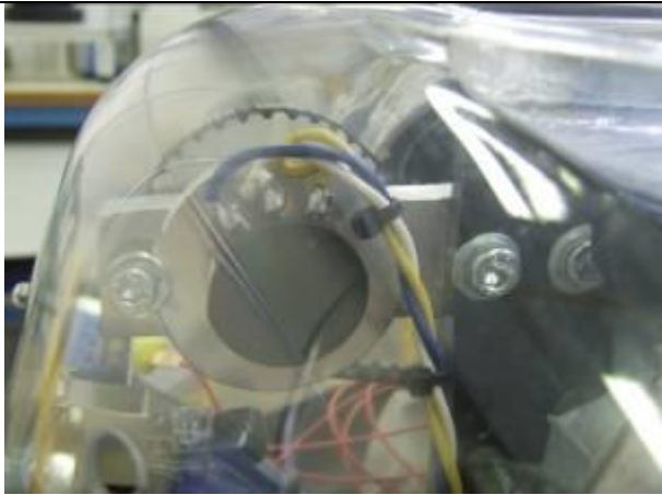
Potentiomètre rotatif (mesure déplacement)
