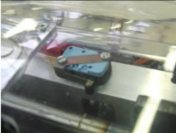
Fin de course de sécurité (déplacement du chariot)
