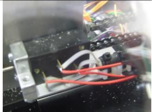
Potentiomètre de mesure de l'écrasement du ressort
