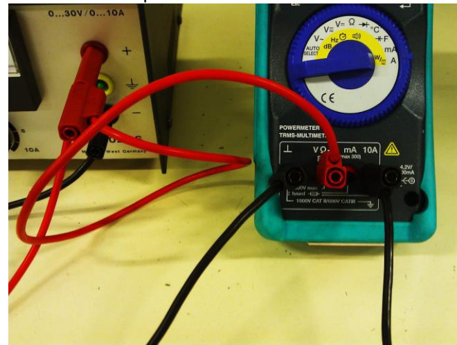
Câblage type de la mesure de puissance / énergie absorbée par un moto-réducteur
